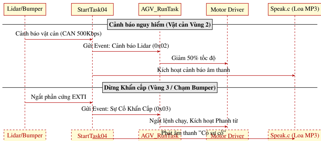
Hình 4.9 Sơ đồ tuần tự luồng giám sát an toàn và xử lý sự cố khẩn cấp.
